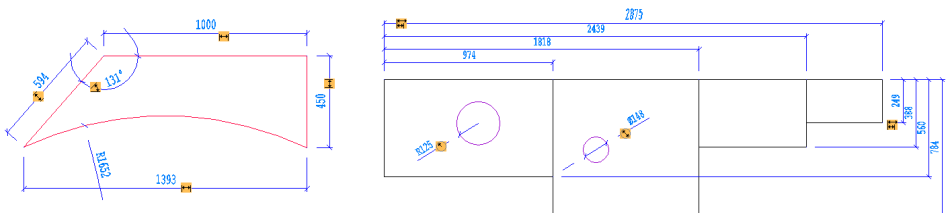
Rys. 91 – przykłady wymiarowania obiektów
