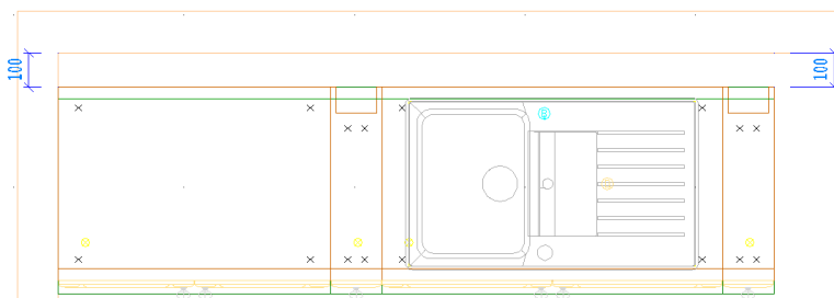
Rys. 178 – szafki wstawione w odległości 100mm od ściany – każda kolejna szafka ma tę samą wartość odsunięcia
