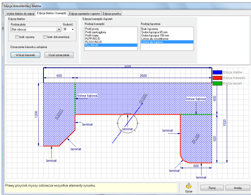
Rys. 255 – oznaczanie kierunku usłojenia blatu
