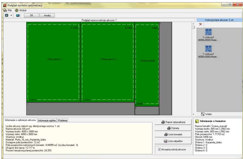
Rys. 541 – przykładowy wzorec rozkroju formatek szafy wewnętrznej w programie CAD Rozkroj v. 3
