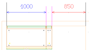
Rys. 180 - brak miejsca na wstawienie szafki szerokości przekraczającej 850mm
