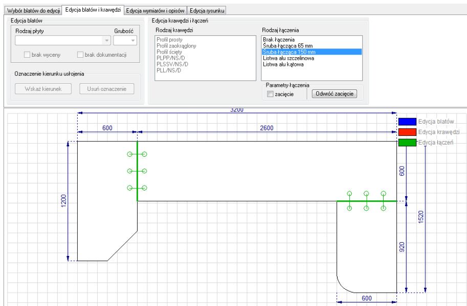
Rys. 253 – wybór łączeń – przykład 1.
