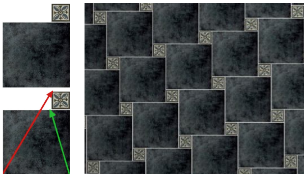
Rys. 397 – tworzenie układu po przekątnej
